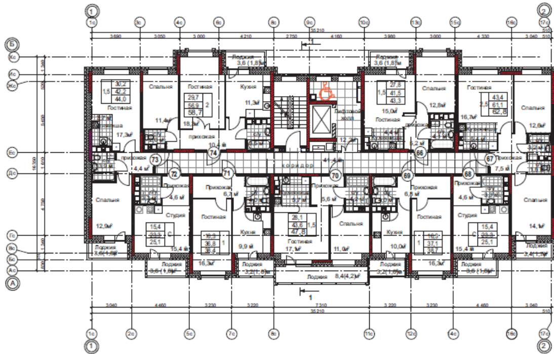
План 3-го этажа 1 секция
